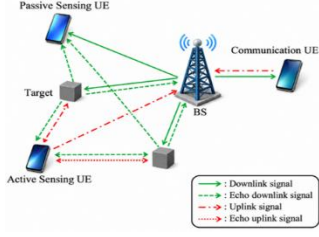
Fig. 5.7. UE-assisted ISAC
